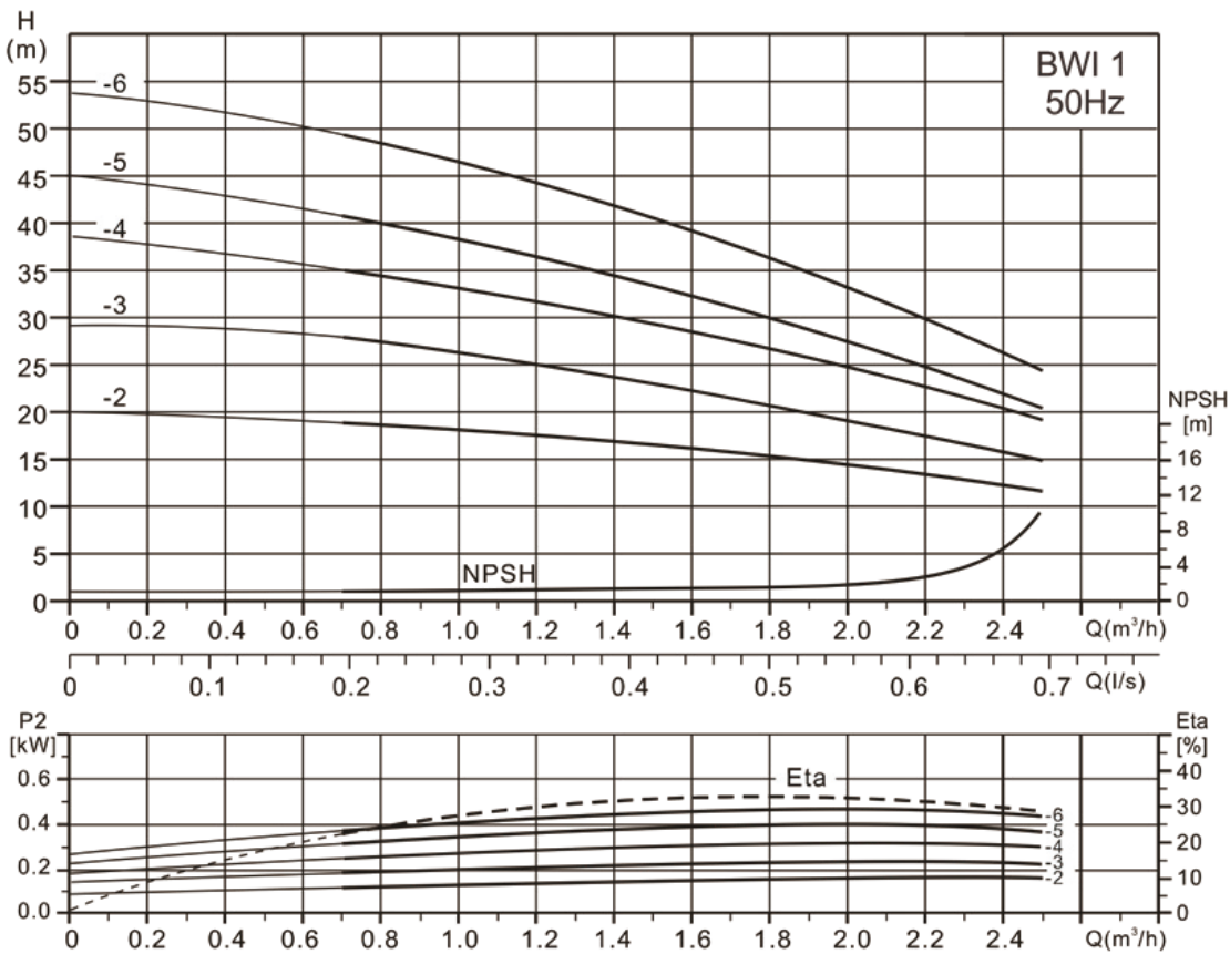
BWI 1性能曲线图
